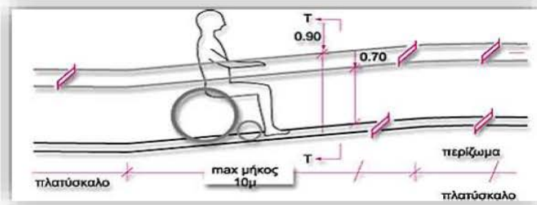
Εικόνα 58. Ράμπα (Υ.Π.ΕΝ., 2020)
