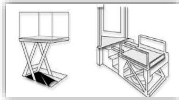
Εικόνα 94. Αναβατόρια κατακόρυφης κίνησης και κλίμακας (Ο.Σ.Κ., 2008)
