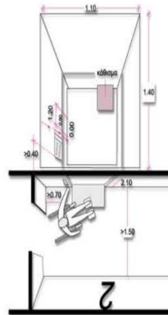
Εικόνα 81. Κάτοψη ανεγκυστήρα (Ο.Σ.Κ., 2008)
