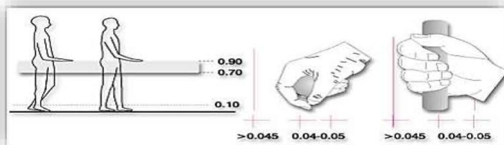
Εικόνα 60. Χειρολισθήρες (Υ.Π.ΕΝ., 2020)
